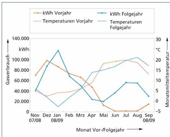
4 – Außentemperaturabhängiger Gasverbrauch vor und nach der Neuinstallation
